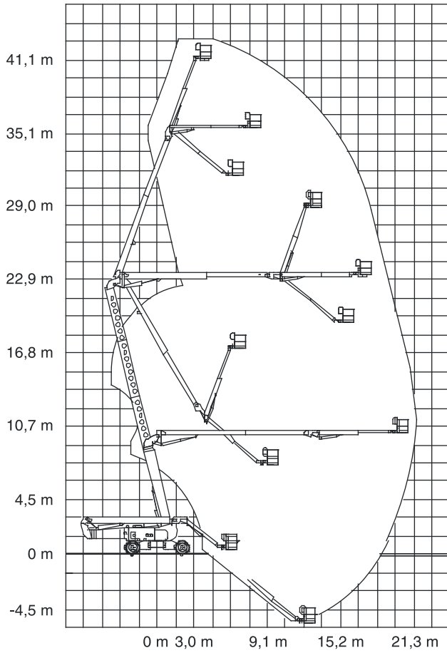
Cuadro de radios de acción del modelo ZX-135/70
