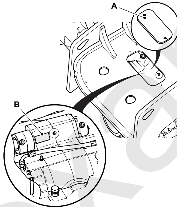
Figura 7. Eje delantero
