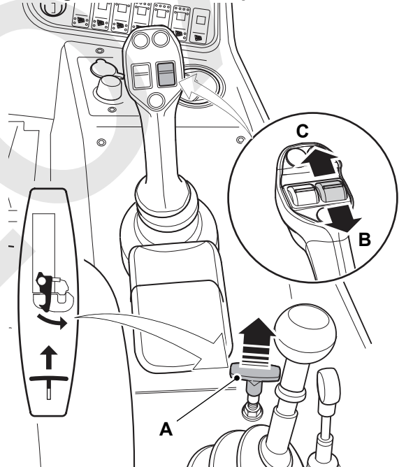
Figura 145. Mando de palanca única
