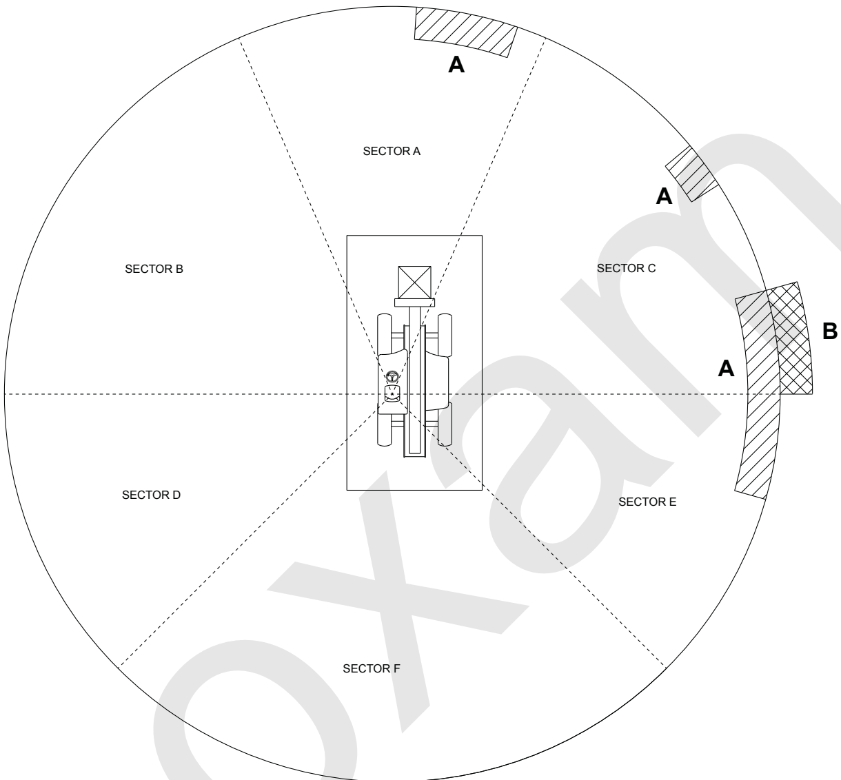
Figura 383. Ocultación de la visibilidad en condición de carga suspendida
